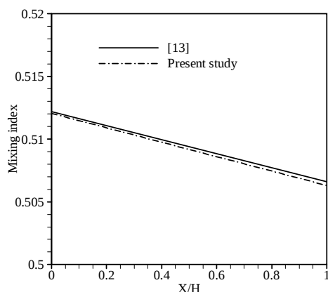
نمودار ۳) مقایسه شاخص اختلاط نسبت به فاصله محوری بی‌بعد به‌ازای k=0.00383 و n=0.9512 در کار حاضر با مرجع [13]
