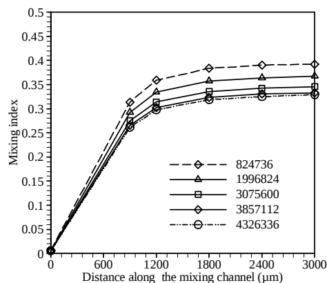
نمودار ۱) شاخص اختلاط در مقاطع عرضی در طول کانال اختلاط به‌ازای شبکه‌بندی‌های مختلف در Re=100 و n=0.75 و k=0.097
