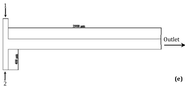
شکل ۱) شماتیک T میکرومیکسرها: (a) هندسه ۱، چندگانه با ورودی‌های ناهم‌راستا در یک صفحه، (b) هندسه ۲، چندگانه با ورودی‌های ناهم‌راستا در دو صفحه، (c) هندسه ۳، چندگانه، (d) هندسه ۴، دوگانه، (e) هندسه ۵
