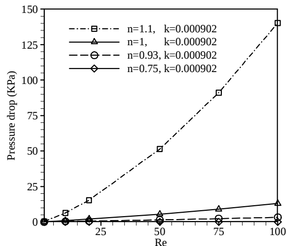
نمودار ۱۹) افت فشار در مقطع عرضی خروجی در محدوده اعداد Re=100 تا Re=10 (هندسه ۱)
