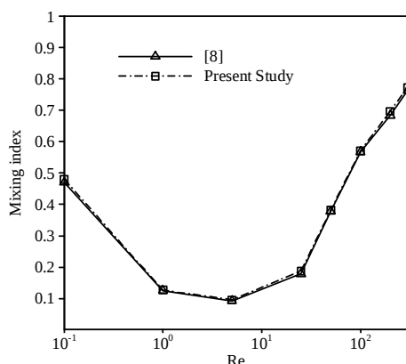
نمودار ۴) مقایسه شاخص اختلاط در محدوده Re=0.1 تا Re=300 به‌ازای سیال با n=1 و k=0.000902 برای کار حاضر و مرجع [8]
