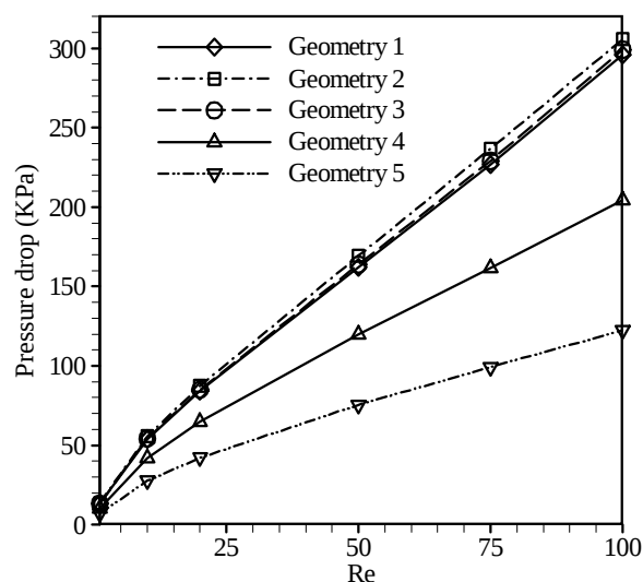
نمودار ۱۴) مقایسه افت فشار در پنج هندسه در محدوده Re=0/1 تا Re=100 به‌ازای k=0/97 و n=0/75
