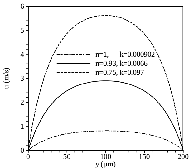
نمودار ۲۰) سرعت کاملاً توسعه‌یافته در دو حالت بی‌بعد و دارای بعد به‌ازای سه سیال مختلف در Re=20 در مقطع خروجی هندسه ۱
