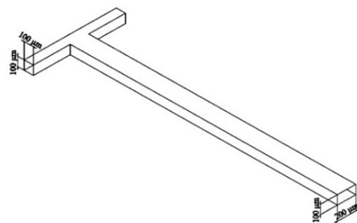
شکل ۱) شماتیک T میکرومیکسرها: (a) هندسه ۱، چندگانه با ورودی‌های ناهم‌راستا در یک صفحه، (b) هندسه ۲، چندگانه با ورودی‌های ناهم‌راستا در دو صفحه، (c) هندسه ۳، چندگانه، (d) هندسه ۴، دوگانه، (e) هندسه ۵
