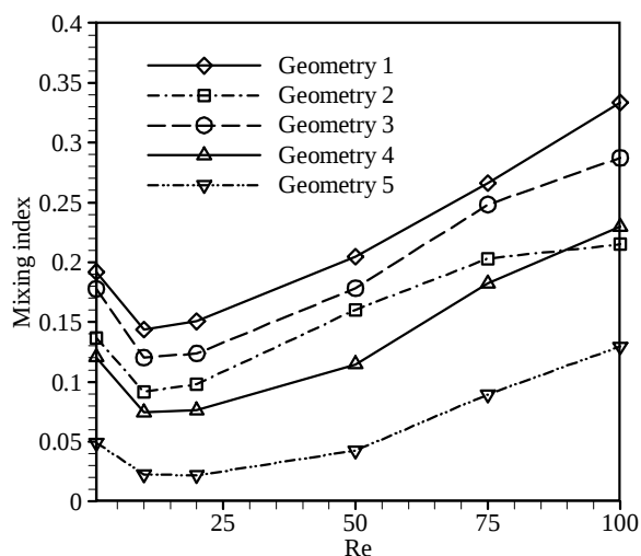
نمودار ۱۱) مقایسه شاخص اختلاط در پنج هندسه در محدوده Re=0 تا Re=100 به‌ازای n=0.93 و k=0.0066 در مقطع عرضی خروجی
