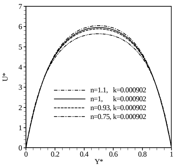
نمودار ۲۱) سرعت کاملاً توسعه‌یافته در دو حالت بی‌بعد و دارای بعد به‌ازای سیال با شاخص‌های توانی مختلف و شاخص پایداری ثابت در Re=20 در مقطع خروجی هندسه ۱
