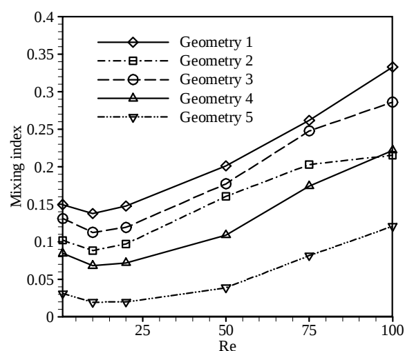
نمودار ۱۳) مقایسه شاخص اختلاط در پنج هندسه در محدوده Re=0 تا Re=100 به‌ازای n=0.75 و k=0.097 در مقطع عرضی خروجی
