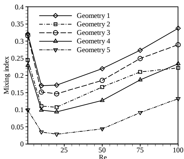
نمودار ۱۶) مقایسه شاخص اختلاط در پنج هندسه در محدوده Re=0 تا Re=100 به‌ازای n=1 و k=0.000902 در مقطع عرضی خروجی
