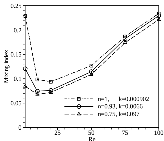
نمودار ۱۲) شاخص اختلاط برای سه سیال مختلف در مقطع عرضی خروجی برای محدوده Re=0 تا Re=100 (هندسه ۴)
