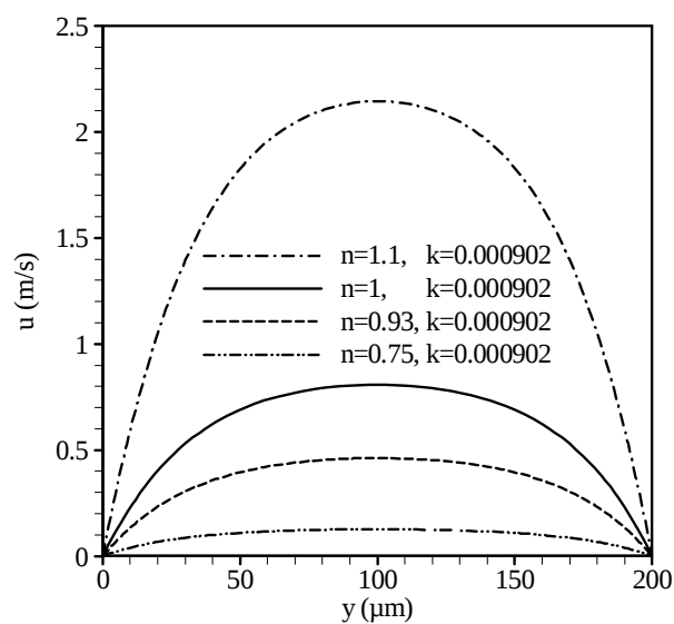
نمودار ۲۱) سرعت کاملاً توسعه‌یافته در دو حالت بی‌بعد و دارای بعد به‌ازای سیال با شاخص‌های توانی مختلف و شاخص پایداری ثابت در Re=20 در مقطع خروجی هندسه ۱
