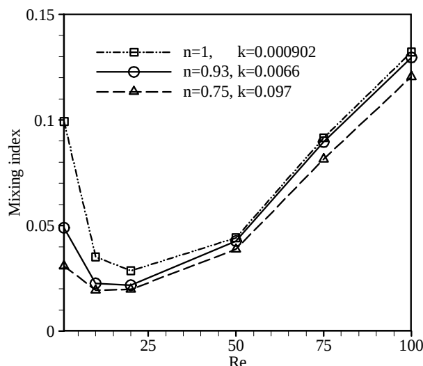
نمودار ۱۴) شاخص اختلاط برای سه سیال مختلف در مقطع عرضی خروجی برای محدوده Re=0 تا Re=100 (هندسه ۵)
