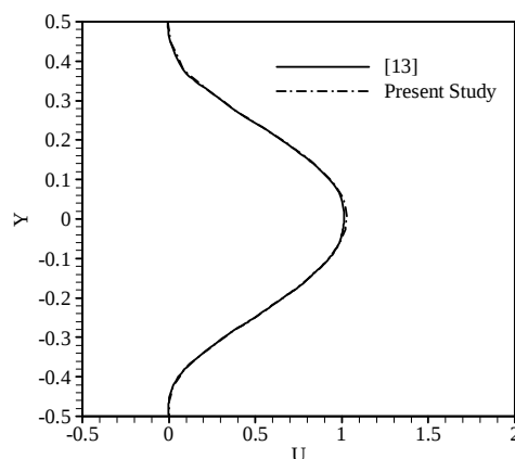
نمودار ۲) سرعت محوری بی‌بعد در نقطه X=0.5 به‌ازای n=0.6161 و k=0.6572 در Re=50 در کار حاضر و مرجع [13]
