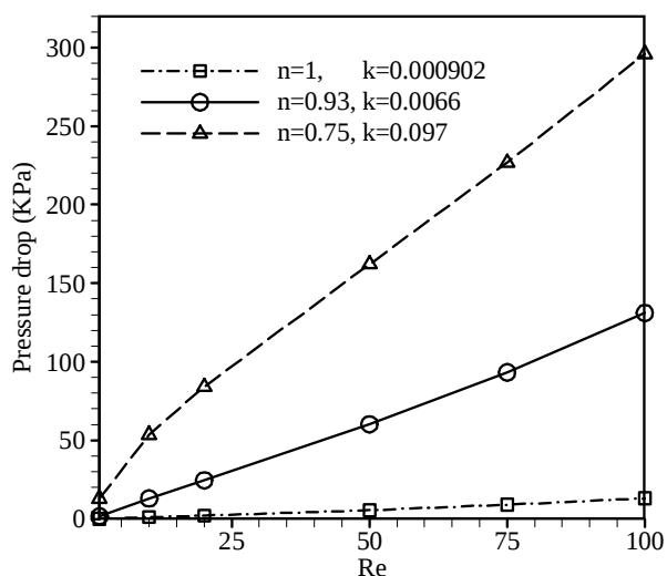
نمودار ۱۵) افت فشار به‌ازای سه سیال مختلف با محدوده Re=0 تا Re=100 در مقطع خروجی (هندسه ۱)
