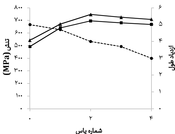
نمودار ۳) تغییرات استحکام تسلیم، استحکام کششی و درصد ازدیاد طول
