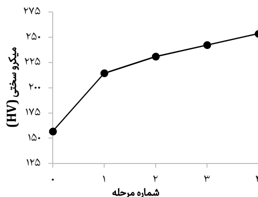
نمودار ۴) تغییرات سختی در نمونه ها به صورت تابعی از تعداد مراحل
