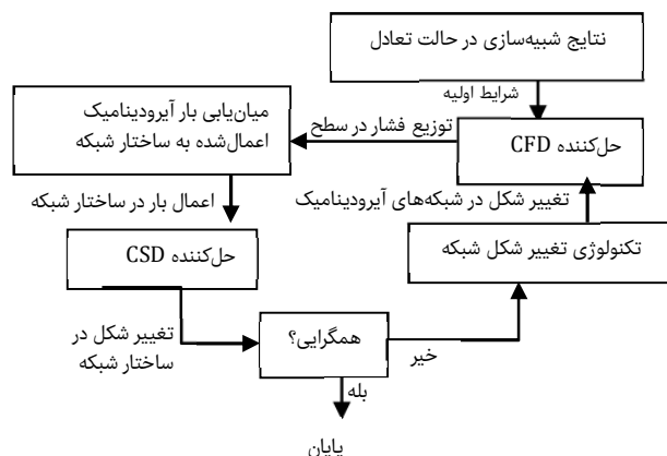
شکل ۷) الگوریتم اتصال دوطرفه نیروهای آیرودینامیک و استاتیک
