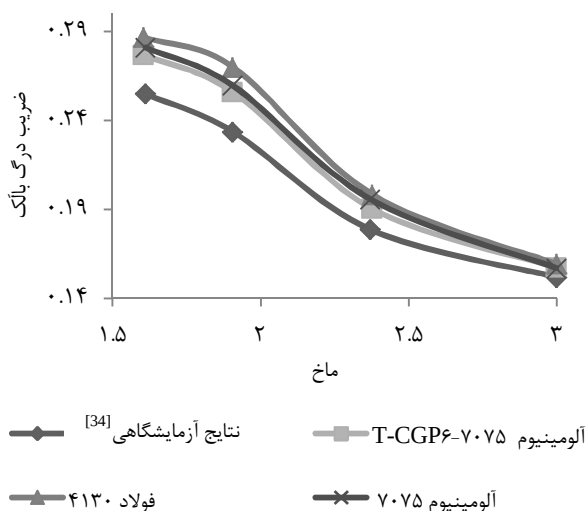
نمودار ۵) مقایسه نمودار ضریب درگ بالک نسبت به ماخ
