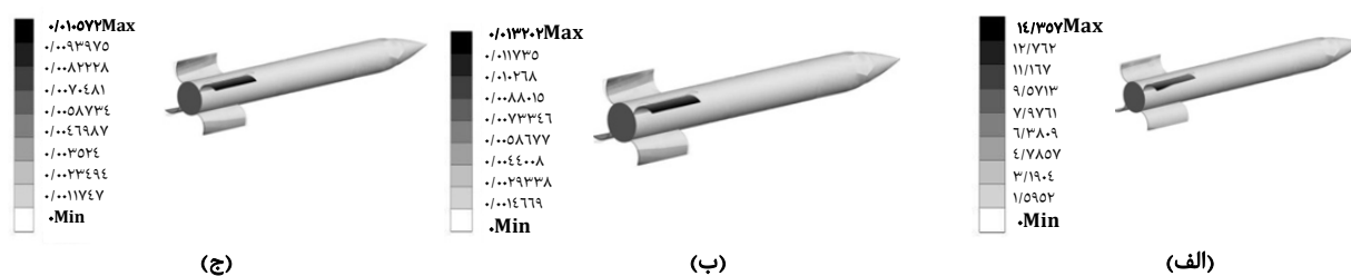
شکل ۱۵ مجموع انحرافات مربوط به بالکها؛ الف) بالک آلومینیوم ۷۰۷۵-T6؛ ب) بالک با جنس آلومینیوم ۷۰۷۵-T6 پرسکاری شیری محدود شده؛ ج) بالک فولاد ۴۱۳۰
