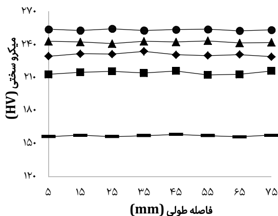
نمودار ۲) مقادیر سختی برحسب فاصله طولی از یک لبه نمونه
