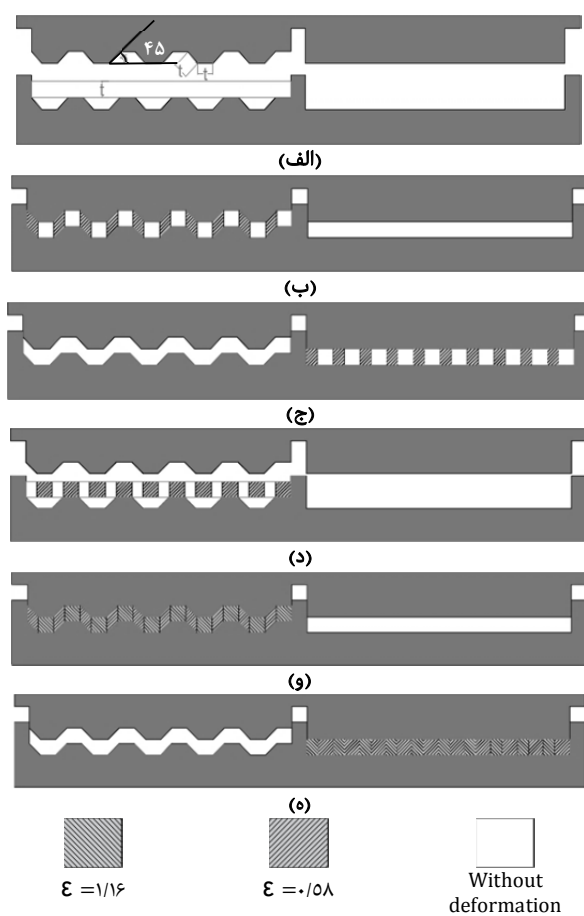
شکل ۲) هندسه مقطع قالب شیاردار و قالب صاف
