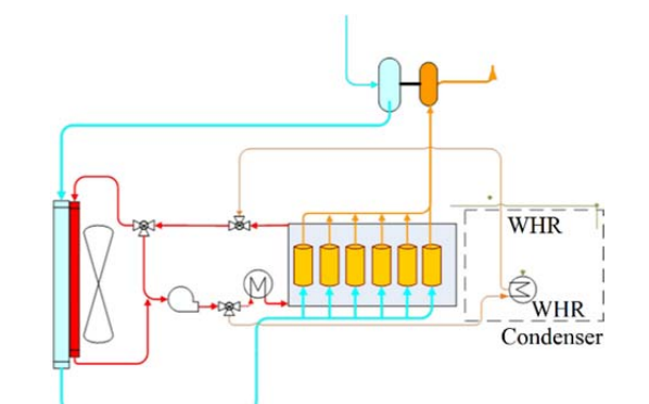
شکل ۷) سرمایه‌ش با ساختار ۲ [۴]
