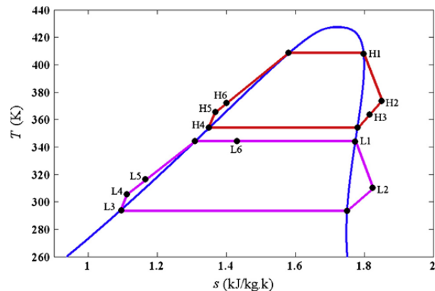
نمودار (۲) دیاگرام دمای آنترنوی سیستم سیکل رانکین ارگانیک دوحلقه [30]
