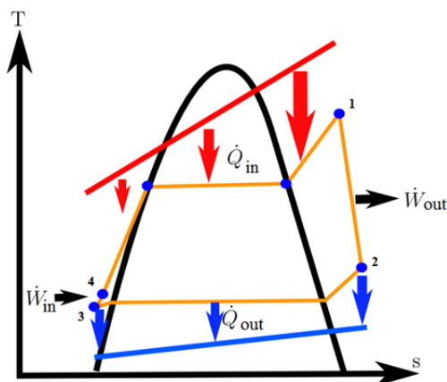
شکل (۱۰) دیاگرام دما آنترپوی سیستم سیکل رانکین ارگانیک
