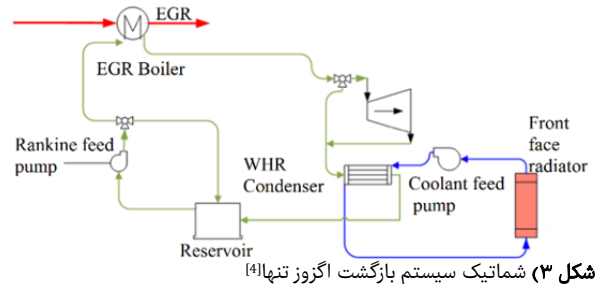
شکل ۳) شماتیک سیستم بازگشت اگزوز تنها [۴]
