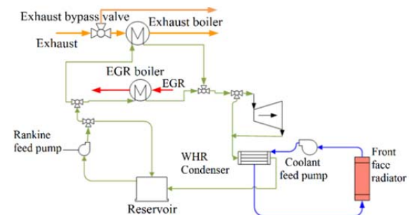
شکل ۴) شماتیک سیستم موازی اگزوز و بازگشت اگزوز [۴]
