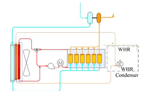
شکل ۶) سرمایه‌ش با ساختار ۱ [۴]
