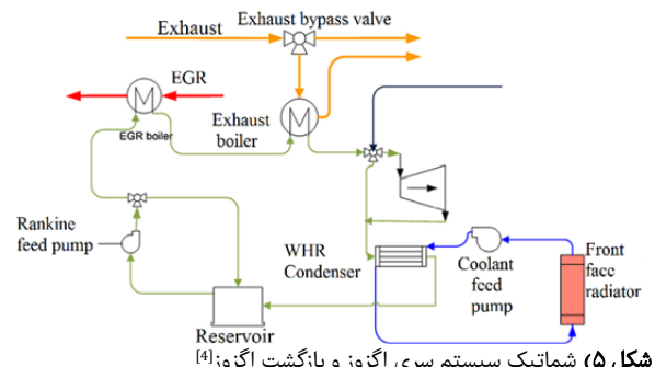
شکل ۵) شماتیک سیستم سری اگزوز و بازگشت اگزوز [۴]
