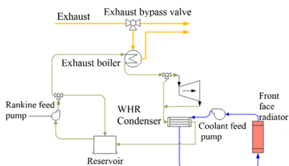
شکل ۲) شماتیک سیستم آگروز تنها [4]
