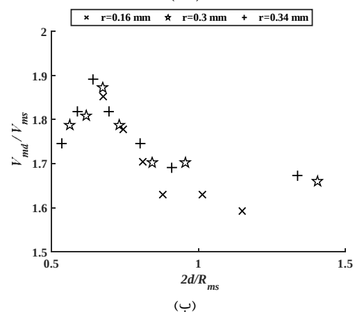
نمودار ۱) تغییرات بیشینه حجم قطرات متصل به فیبرهای موازی با فاصله فیبرها؛ الف) شمای تغییر شکل قطره روی فیبر با شعاع ۰.۳۴ میلی‌متر، ب) تغییرات حجم بیشینه بی‌بعد برحسب فاصله در فیبرها با شعاع‌های مختلف
