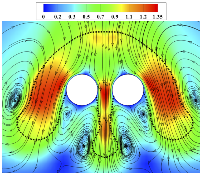
شکل ۴) خطوط مسیر و کانتور سرعت بر صفحه دوبعدی در برخورد قطره با شعاع ۱.۴ میلی‌متر بر فیبر با شعاع ۰.۳۵ میلی‌متر با سرعت برخورد یک‌متر در ثانیه؛ فاصله بین مرکز دو فیبر برابر یک میلی‌متر است.
