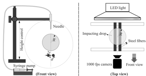
شکل ۱) شمای نحوه انجام آزمایش
