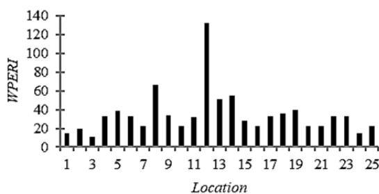
نمودار ۷) مقادیر شاخص نرخ انرژی بر پایه تبدیل موجک بسته‌ای در ترک در ۱/۲ دهانه با عمق ۸۰٪
