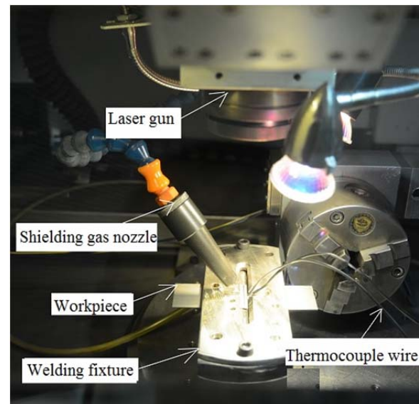
شکل ۲) آماده‌سازی بستر آزمایش و نمایی از فیکسچر جوشکاری
