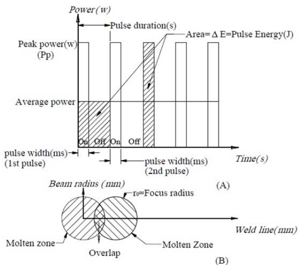
شکل ۸ شماتیک جوشکاری لیزر پالسی
