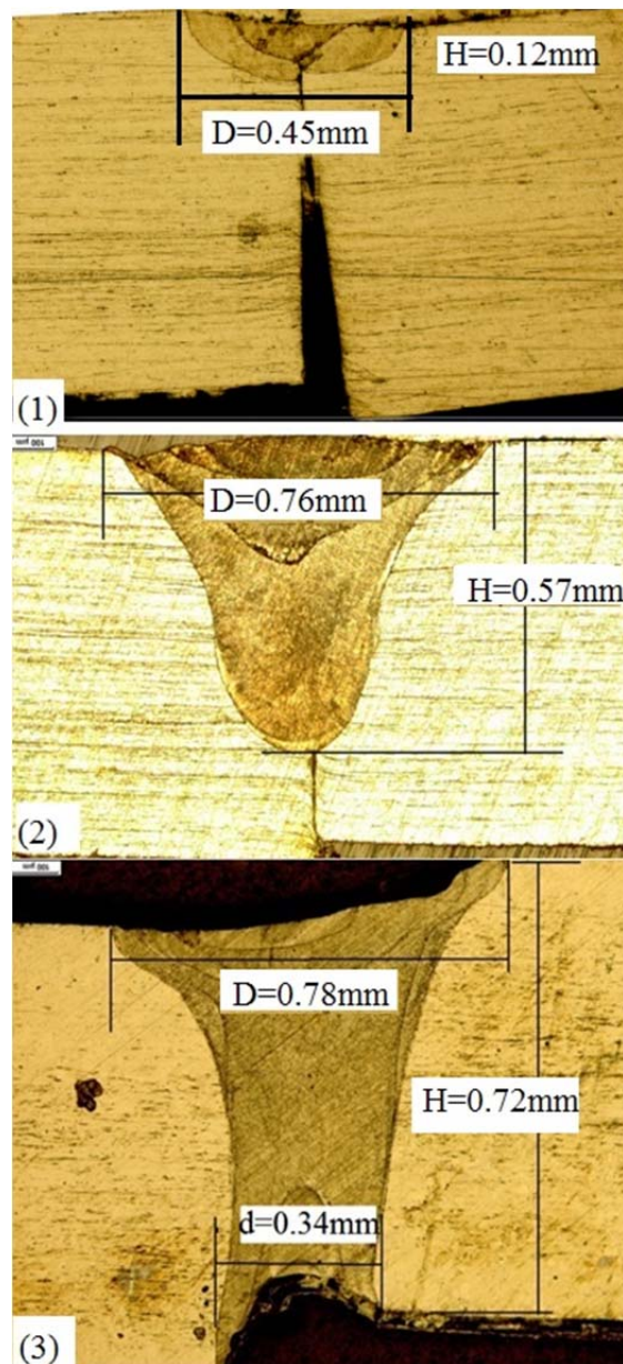
شکل ۱۳) ابعاد هندسه جوش در سه آزمایش تجربی
