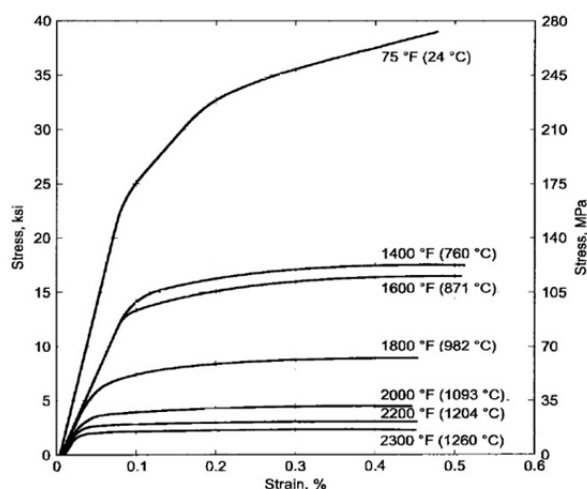
نمودار ۱) نمودار تنش- کرنش مهندسی در دماهای مختلف برای آلیاژ AISI316L [15]
