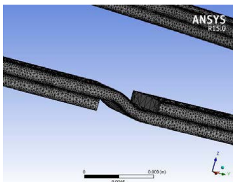
شکل ۶) مدل آب‌بند مکانیکی لامینار مش‌بندی شده
