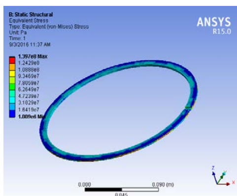
شکل ۱۱) توزیع تنش (وون‌میسز) آب‌بند مکانیکی لامینار در شرایط بارگذاری استاتیکی
