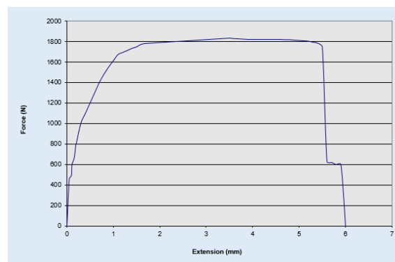
نمودار ۲) نمودار نیرو- جابه‌جایی مفتول نوردشده
