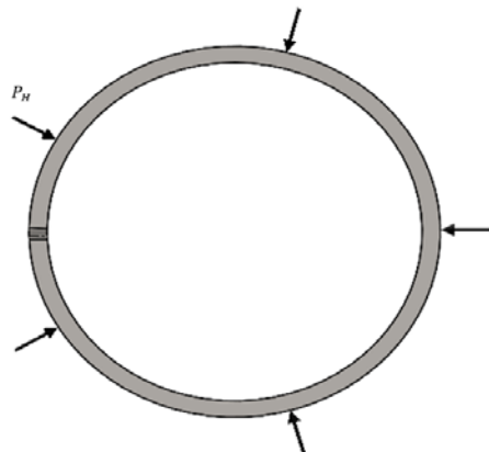
شکل (۲) چگونگی اعمال فشار ناشی از سفت‌کردن پوسته یاتاقان روی آب‌بند مکانیکی لامینار P_H
