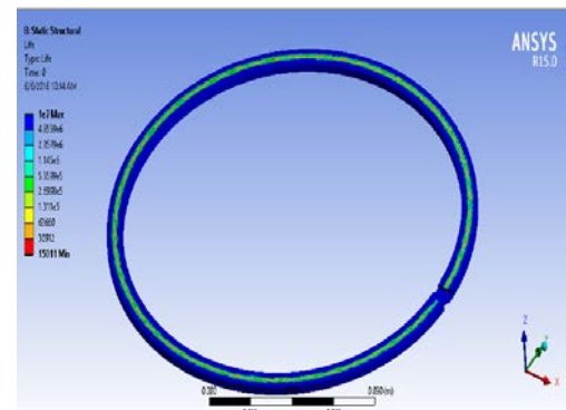
شکل ۱۴) عمر آب‌بند مکانیکی لامینار در شرایط بارگذاری خستگی
