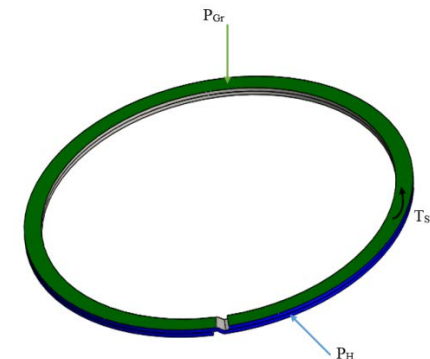
شکل (۱) مجموعه نیروهای وارده بر آب‌بند مکانیکی لامینار
