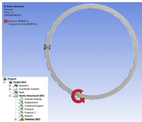
شکل ۷) مدل آب‌بند پس از اعمال شرایط مرزی و بارگذاری استاتیک
