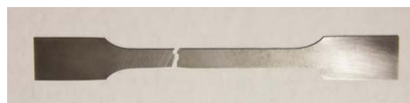
شکل ۹) نمونه آزمون کشش مفتول نوردشده پس از شکست
