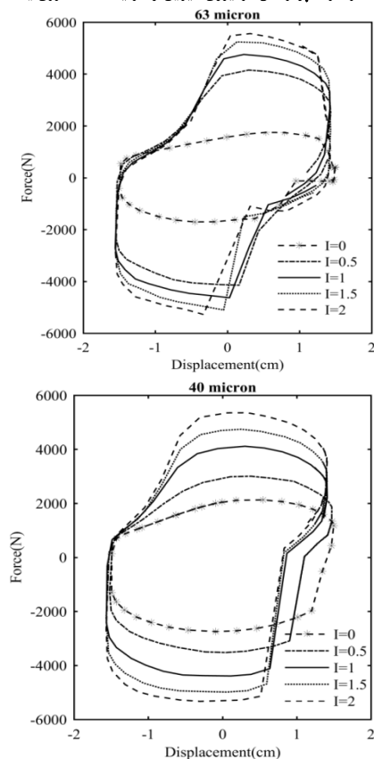
نمودار ۳) منحنی‌های تست هسترزیس نیرو- جابه‌جایی در فرکانس ۰/۲۵ هرتز برای سیال ۴۰ و ۶۳ میکرون
