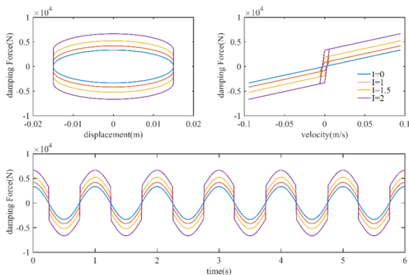
نمودار ۱) شبیه‌سازی MR دمپر براساس معادلات غیرخطی بینگهام
