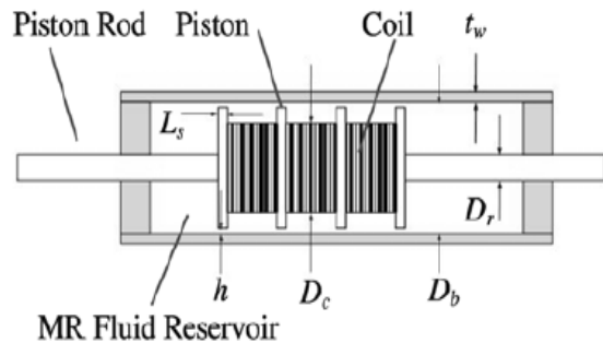
شکل ۲) شماتیک دمپر دوسرمتحرک با سه کوئل الکتریکی
