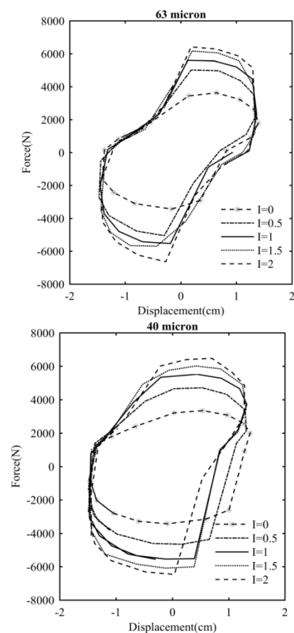
نمودار ۴) منحنی‌های تست هسترزیس نیرو- جابه‌جایی در فرکانس ۰/۵ هرتز برای سیال ۴۰ و ۶۳ میکرون
