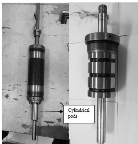
شکل ۳) پیستون و دمپر مگنتورئولوژیکال؛ الف) پیستون، ب) دمپر مگنتورئولوژیکال
