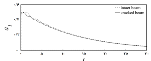
نمودار ۸) تغییرات a_1 در ارتعاشات آزاد تیر سالم و تیر با ترک در موقعیت نسبی ۰/۶ و عمق نسبی ۰/۴، ضریب میرایی مودال ۰/۰۰۵
