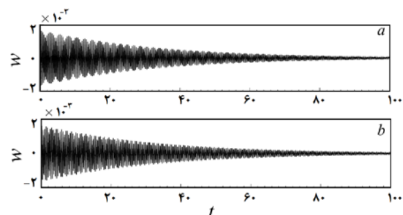
نمودار ۱) پاسخ ارتعاشات آزاد تیر: (a) در حالت سالم، (b) با یک ترک با عمق نسبی ۰/۵ در موقعیت نسبی ۰/۶
