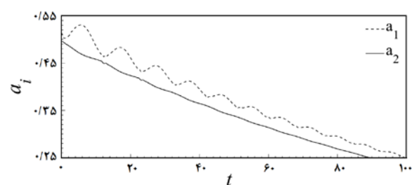
نمودار ۳) تغییرات دامنه آنی مدهای ارتعاشی تیر سالم در لحظات اولیه ارتعاش آزاد
