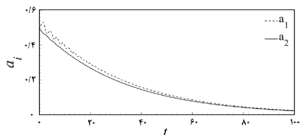
نمودار ۲) دامنه آنی مدهای ارتعاشی اول و دوم تیر سالم
