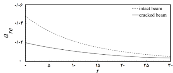
نمودار ۷) تغییرات a_{re} در ارتعاشات آزاد تیر سالم و تیر با ترک در موقعیت نسبی ۰/۶ و عمق نسبی ۰/۴، ضریب میرایی مودال ۰/۰۰۲
