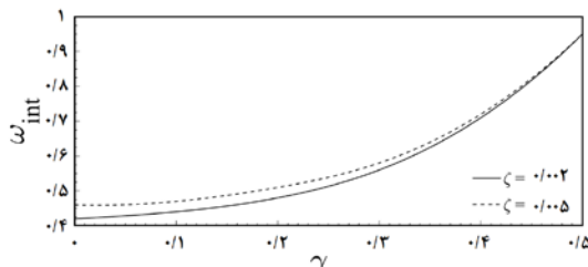
نمودار ۱۰) تغییرات \omega_{int} در تیر با ترک در موقعیت l_1=0.6 در برابر عمق نسبی ترک به ازای ضرایب میرایی مودال ۰/۰۰۲ و ۰/۰۰۵
