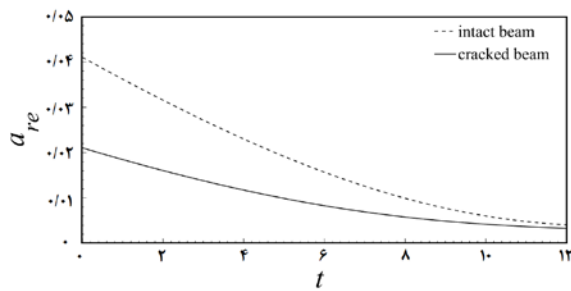
نمودار ۹) تغییرات a_{re} در ارتعاشات آزاد تیر سالم و تیر با ترک در موقعیت نسبی ۰/۶ و عمق نسبی ۰/۴، ضریب میرایی مودال ۰/۰۵
