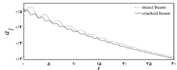
نمودار ۶) تغییرات a_1 در ارتعاشات آزاد تیر سالم و تیر با ترک در موقعیت نسبی ۰/۶ و عمق نسبی ۰/۴، ضریب میرایی مودال ۰/۰۰۲
