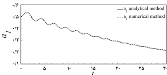
نمودار ۴) دامنه آنی مود ارتعاشی اول به‌دست‌آمده از روش‌های تحلیلی و عددی
