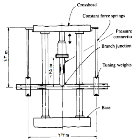
شکل ۱) دستگاه آزمون سهرای تحت خمش صفحه‌ای [10]
