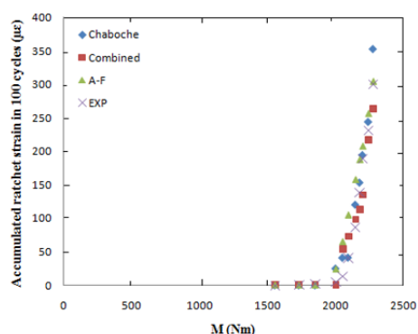
نمودار ۵) تغییر شکل‌های پیش‌رونده به‌دست‌آمده از نتایج تجربی و عددی برای نمونه BSS3 برحسب گشتاور
