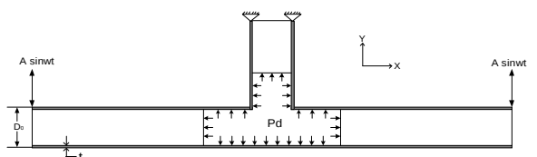
شکل ۲) نمونه لوله سهرای
