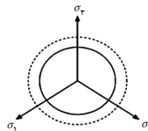
شکل ۳) مدل سخت شوندهگی ایزوتروپیک
