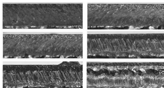
شکل ۳) چند نمونه از سطح دیواره برش در شرایط مختلف برش پلاسما
