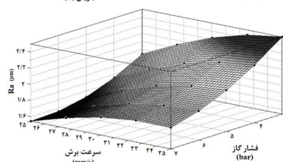
نمودار ۲) تأثیر پارامترهای جریان و فشار گاز و همچنین تأثیر جریان و سرعت پیشروی بر زبری سطح
