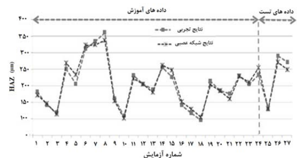
نمودار ۵) مقایسه بین داده‌های تجربی و داده‌های پیش‌بینی برای منطقه متأثر از حرارت
