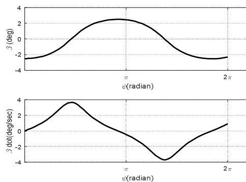
نمودار ۱۷) تغییرات زاویه فلپینگ و نرخ آن در پرواز کروز با فرض داشتن آفست پره e = 0.4 (مقادیر بزرگ زاویه فلپینگ)
