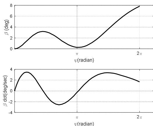
نمودار ۷) تغییرات زاویه فلپینگ و نرخ آن در پرواز کروز با فرض e = 0.15 و R = 15
