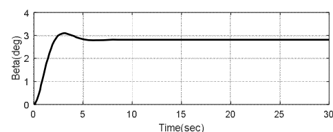
نمودار ۱۴) تغییرات زمانی زاویه فلپینگ و نرخ آن در پرواز هاور با فرض داشتن آفست پره
