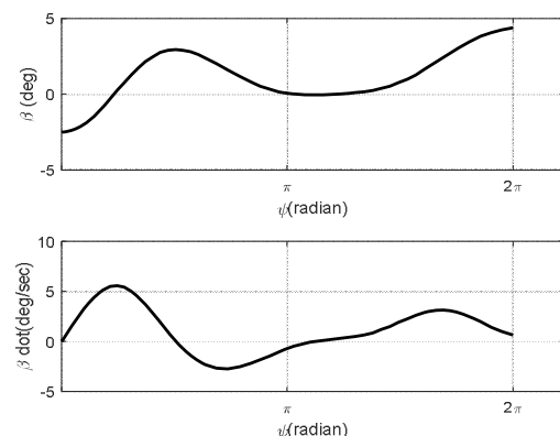
نمودار ۲) تغییرات زاویه فلپینگ و نرخ آن در پرواز کروز با فرض e = ۰ و \mu = ۱ و \alpha = ۱ radian
