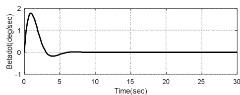
نمودار ۱۵) تغییرات زمانی زاویه فلپینگ و نرخ آن در پرواز هاور با فرض نداشتن آفست پره
