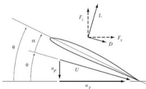
شکل ۴) نیروها و سرعت‌های سطح مقطع پره روتور [22]
