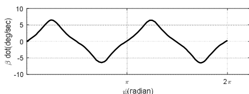
نمودار ۱۶) تغییرات زاویه فلپینگ و نرخ آن در پرواز کروز با فرض داشتن آفست پره e = 0.15 (مقادیر بزرگ زاویه فلپینگ)
