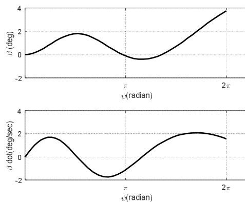
نمودار ۶) تغییرات زاویه فلپینگ و نرخ آن در پرواز کروز با فرض e = 0.15 و R = 5
