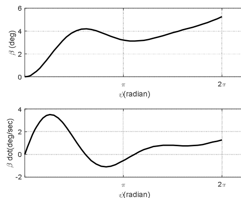
نمودار ۴) تغییرات زاویه فلپینگ و نرخ آن در پرواز کروز با فرض e = 0.5 و \theta_{twist} = 0
