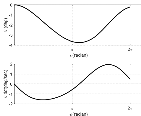
نمودار ۵) تغییرات زاویه فلپینگ و نرخ آن در پرواز کروز با فرض e = 0.5 و \theta_{twist} = 0
