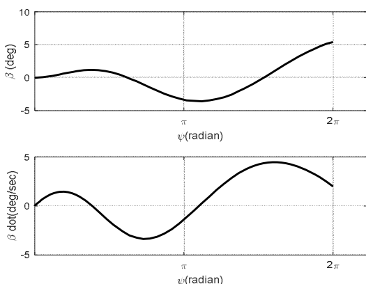
نمودار ۸) تغییرات زاویه فلپینگ و نرخ آن در پرواز کروز با فرض e = 0.15 و \theta_{twist} = 9
