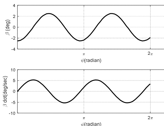
نمودار ۱۹) تغییرات زاویه فلپینگ و نرخ آن در پرواز کروز با فرض داشتن آفست پره e = 0.4 (مقادیر کوچک زاویه فلپینگ)
