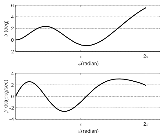
نمودار ۹) تغییرات زاویه فلپینگ و نرخ آن در پرواز کروز با فرض e = 0 تحت اثر گشتاور وزن پره
