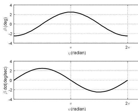
نمودار ۳) تغییرات زاویه فلپینگ و نرخ آن در پرواز کروز با فرض e = 0.15 و Nb = 2 و \alpha = 1 radian
