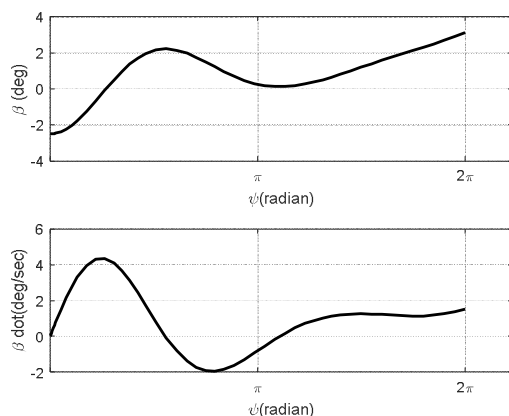
نمودار ۱) تغییرات زاویه فلپینگ و نرخ آن در پرواز کروز با فرض e = ۰ و \mu = ۰/۵ و \alpha = ۱ radian
