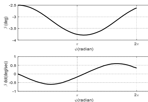
نمودار ۱۸) تغییرات زاویه فلپینگ و نرخ آن در پرواز کروز با فرض نداشتن آفست پره e = 0 (مقادیر بزرگ زاویه فلپینگ)
