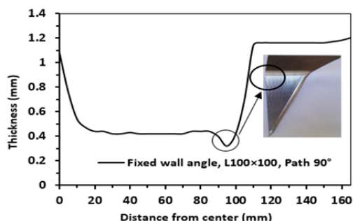
نمودار ۸) توزیع ضخامت از هرم ناقص با ابعاد قاعده ۱۰۰×۱۰۰ میلی‌متر مربع، زاویه جداره ثابت ۶۷ درجه و جهت برش ۹۰ درجه
