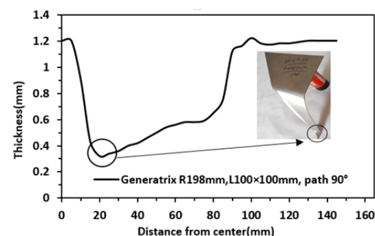
نمودار ۱۱) توزیع ضخامت از هرم ناقص با ابعاد قاعده ۱۰۰×۱۰۰ میلی‌متر مربع، با زاویه جداره متغیر با شعاع ۱۹۸ میلی‌متر و ارتفاع ۱۲۲ میلی‌متر در جهت برش ۹۰ درجه
