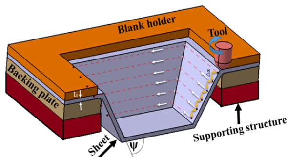
شکل ۱) شماتیک کلی شکل‌دهی تدریجی تک‌نقطه‌ای هرم ناقص
