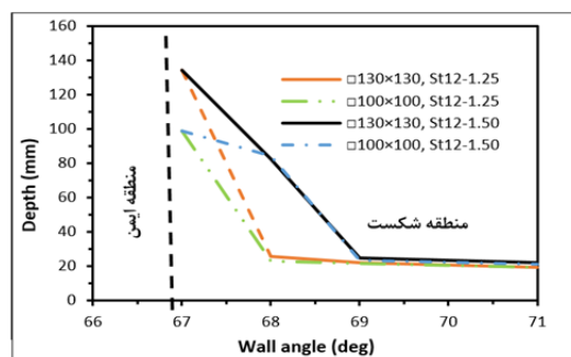
نمودار ۹) شکل‌دهی فرآیندی تجربی ورق St12 در شکل‌دهی تدریجی تک‌نقطه‌ای هرم ناقص با زاویه جداره ثابت
