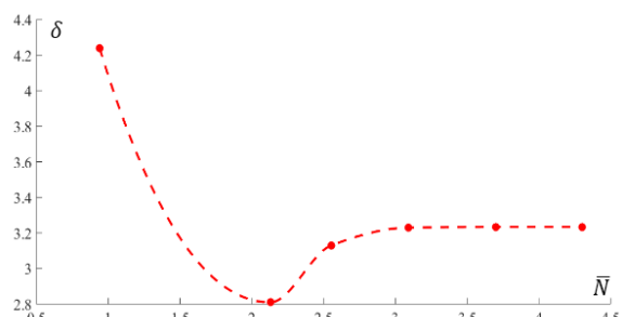
نمودار ۳) ضخامت صفحه مشترک فازی برحسب پارامتر \bar{N}
