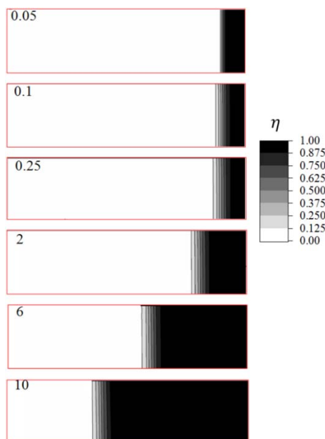
شکل ۱) مراحل انتشار صفحه فازی مشترک برای زمان‌های مختلف در \bar{\theta} = 0.53
