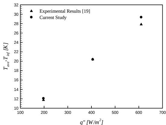
نمودار (۱) مقایسه نتایج دمایی به دست آمده در این تحقیق با مرجع [۱۹]
