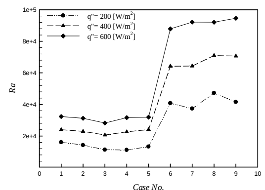
نمودار ۱۳) نمودار عدد بی‌بعد رایلی برای شارهای حرارتی مختلف
