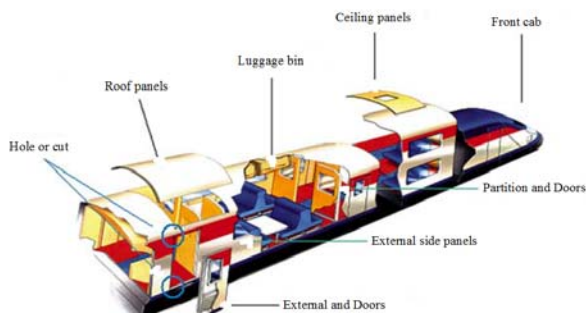
شکل ۱) قسمت‌های کامپوزیتی به کار رفته در قطار پرسرعت [1]
