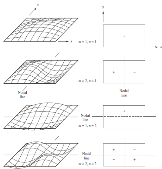
شکل (۵) شکل مدهای یک ورق مستطیلی با تکیه‌گاه‌های ساده [18]
