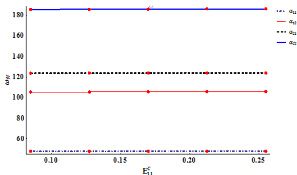
نمودار (۵) تأثیر تغییرات مدول هسته در جهت X بر فرکانس
