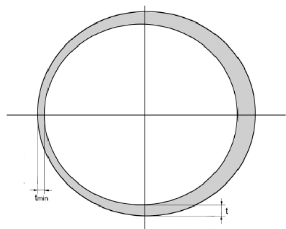
شکل ۳ خارج از مرکزی لوله [3]
