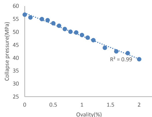
نمودار ۶) تغییرات فشار مچالگی برحسب تغییر اوالیته
