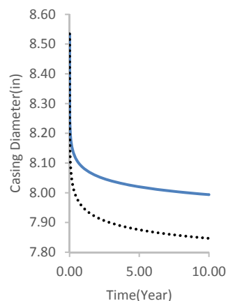
نمودار ۴) تغییرات قطر لوله جداری ایجادشده در لوله جداری چاه مورد نظر با در نظر گرفتن ۲٪ خارج از مرکزی و بیضی‌بودن بر اثر خزش سنگ نمک سازند گچساران
