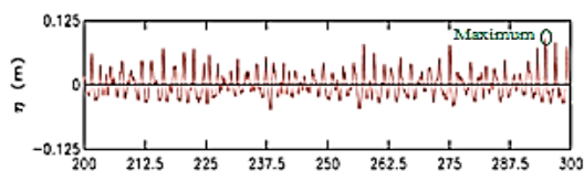
نمودار ۲) تاریخچه زمانی پروفیل سطح آب در آزمایشگاه در اثر موج تصادفی با ارتفاع موج مشخصه ۱/۰ متر و پریود ۲ ثانیه [16]
