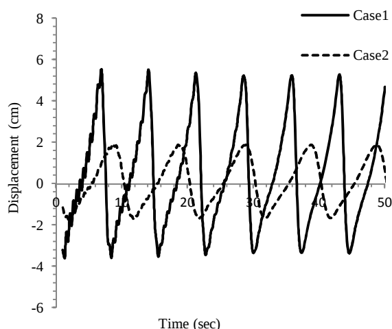
نمودار ۹) تاریخچه زمانی جابجایی حداکثر مونوپایل تحت تئوری استوکس مرتبه ۵ برای Case2 و Case1
