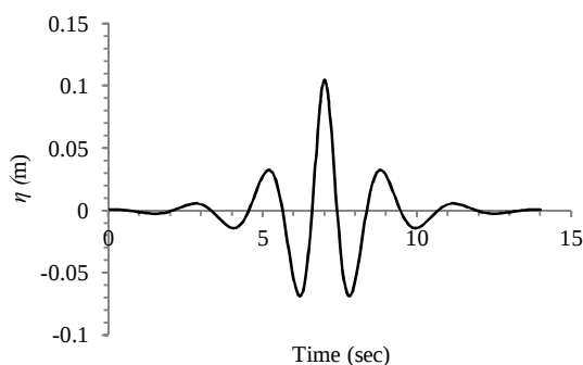
نمودار ۳) تاریخچه زمانی تراز سطح آب در تئوری موج نو برای ارتفاع موج مشخصه ۱/۰ متر و پریود ۲ ثانیه
