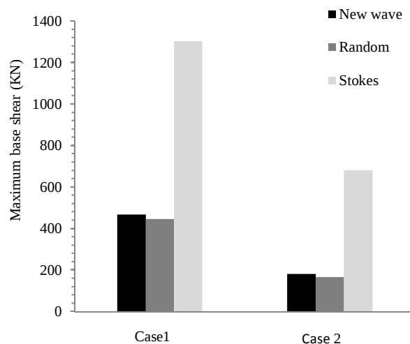
نمودار (۱۱) مقایسه برش پایه حداکثر مونوپایل در تئوری‌های موج نو، تصادفی خطی و استوکس مرتبه ۵
