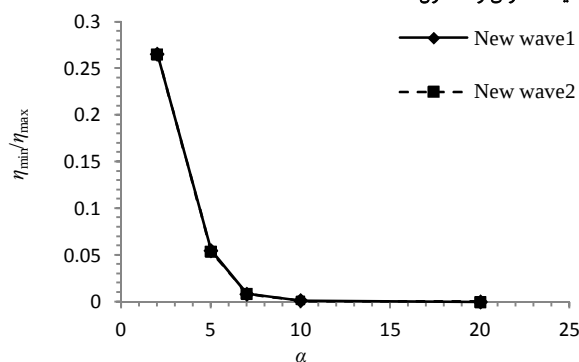
نمودار ۴) تعیین مدت زمان شبیه‌سازی تحت تئوری موج نو
