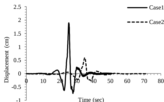
نمودار ۷) تاریخچه زمانی جابجایی حداکثر مونوپایل تحت تئوری موج نو برای Case1 و Case2
