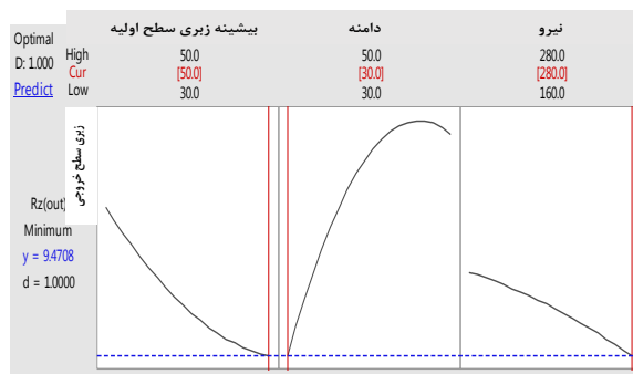
نمودار ۱۰) شرایط بهینه در صیقل‌کاری به کمک نوسانات فراصوتی
