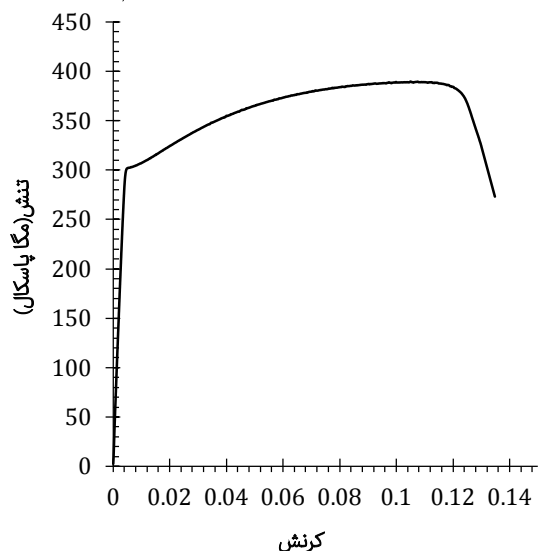
نمودار ۱) نمودار تنش و کرنش به دست آمده از آزمون کشش برای آلیاژ Al6061-T6
