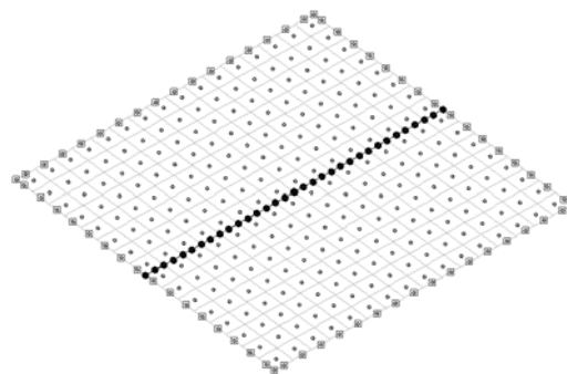
شکل ۱۱ شبکه نقاط کنترلی برای ورق تقویت‌شده با یک تقویت‌کننده مستقیم مرکزی
