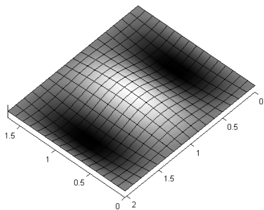
شکل ۱۵ مود کمانشی ورق استحکام‌یافته با دو تقویت‌کننده مستقیم
