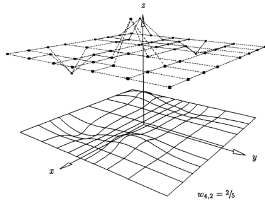
شکل ۲ نمونه‌ای از شبکه نقاط کنترلی و سطح نریز مربوط به آن [35]
