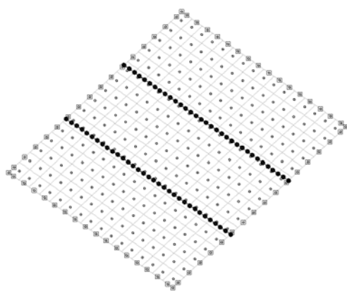
شکل ۱۴ شبکه نقاط کنترلی برای ورق تقویت‌شده با دو تقویت‌کننده مستقیم
