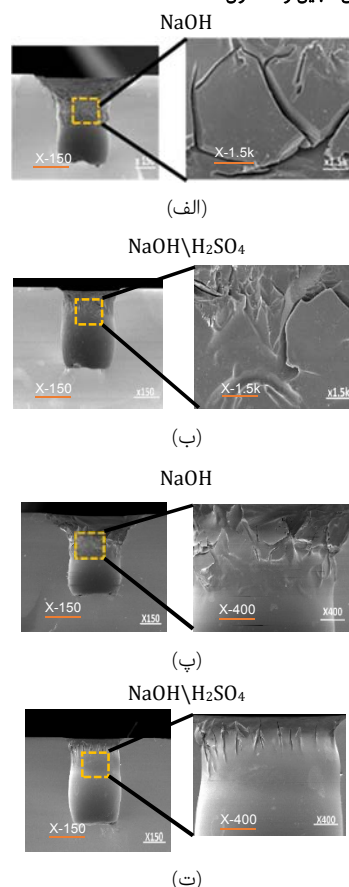
شکل ۹) تصاویر میکروسکوپ الکترونی روبشی از سطوح سوراخ در دمای ۴۵°C
