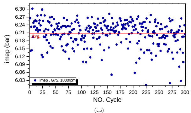
نمودار ۳) تغییرات IMEP سیکل‌های پشت سر هم برحسب شماره ترتیب وقوع سیکل در آوانس بهینه برای (الف) G100 و (ب) G75
