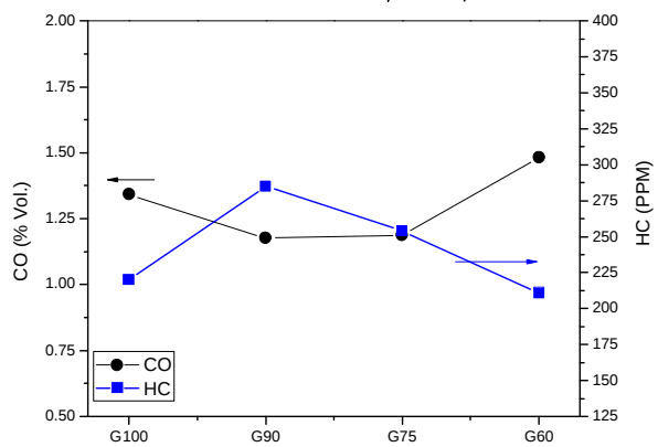
نمودار ۹) تغییرات CO، HC برحسب درصد حضور بنزین در مخلوط
