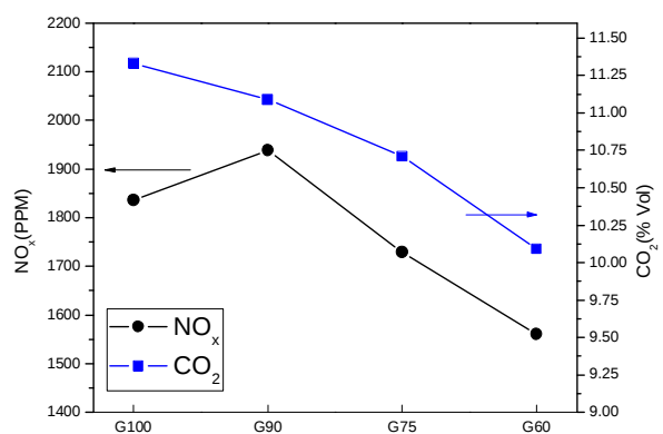
نمودار ۱۰) تغییرات NO x و دمای گازهای حاصل از احتراق برحسب درصد حضور بنزین در مخلوط
