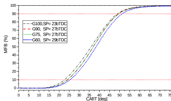
نمودار ۹) تغییرات کسر جرمی سوخته برحسب زاویه میل‌لنگ از موقعیت جرقه به ازای درصد حضور بنزین در ترکیب دو سوخت
