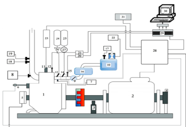
شکل ۱) نمایی از بستر آزمایش و تعلیقات مربوطه
