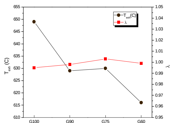
نمودار ۸) تغییرات \lambda و دمای گازهای خروجی موتور در حالت مختلف ترکیب دو سوخت
