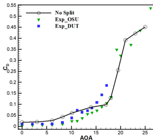
نمودار ۳) اعتبارسنجی مدل حل عددی، مقایسه ضریب پسا در حل عددی پژوهش حاضر (No Split) و نتایج تجربی
