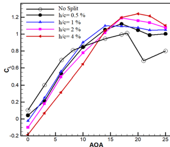
نمودار ۶) مقایسه ضرایب برآی ایرفویل خانواده S809-4090
