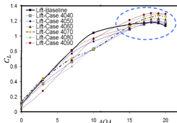
نمودار (۱) اثر ایجاد شکاف در ایرفویل S809 بر ضریب برآ در زوایای حمله مختلف که تأثیر مثبت آن مشخص شده است [7]
