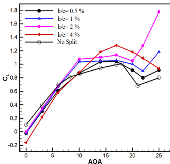
نمودار ۴) مقایسه ضرایب برای ایرفویل خانواده S809-3090
