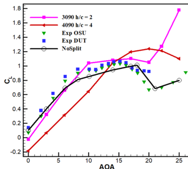
نمودار ۸ نمودار مقایسه ضرایب نیروی برآ برای ضخامت های بهینه شکاف در ایرفویل های خانواده های S809-4090 و S809-3090
