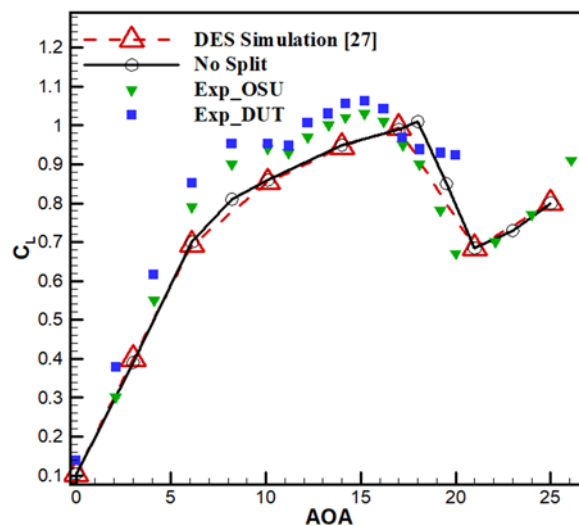
نمودار ۲) اعتبارسنجی مدل حل عددی، مقایسه ضریب برآ در حل عددی پژوهش [26]، پژوهش حاضر (No Split) و نتایج تجربی
