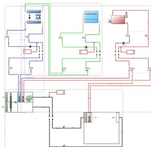
شکل ۴) جزئیات مدارهای مدل‌سازی شده چیلرها در نرم‌افزار
