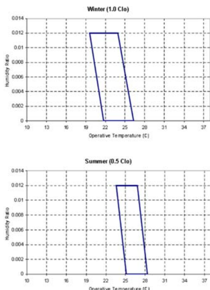
نمودار ۱) نمودار آسایش در استاندارد ASHRAE 55 در زمستان (بالا) و تابستان (پایین)
