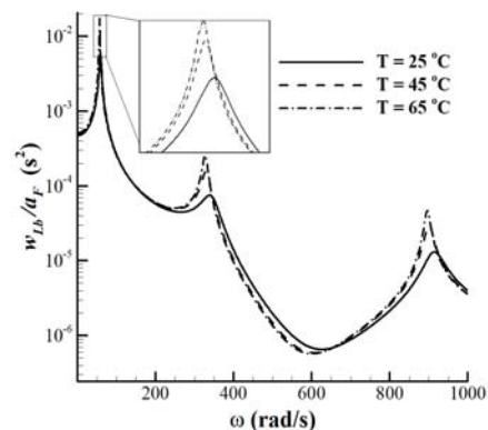
نمودار ۵) پاسخ فرکانسی در انتهای تیر برای سه دمای مختلف
