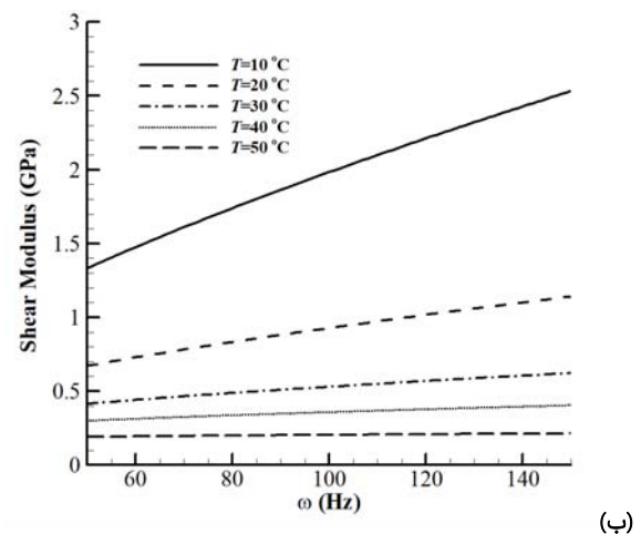
نمودار ۱) تغییرات مدول برشی به دست آمده از رابطه ۸، الف) با دما برای فرکانس‌های مختلف و ب) با فرکانس برای دماهای مختلف
