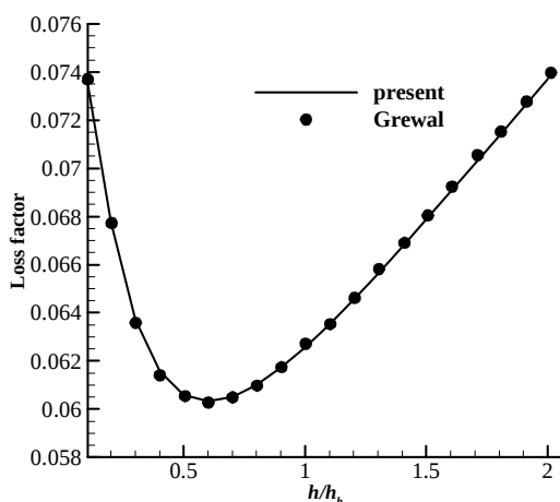
نمودار ۲) مقایسه میرایی محاسبه شده برای تیر با لایه میرایی مقید سرتاسری با نتایج مطالعه گروال [17]
