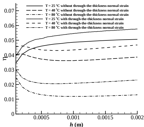
نمودار ۱۰) اثر حذف کرنش راستای ضخامت در تغییرات میرایی با ضخامت هسته به‌ازای مقادیر مختلف دما
