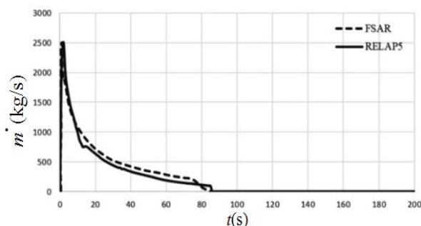
نمودار ۱) میزان دبی شکستگی از سمت اتصال به مولد بخار دوم
