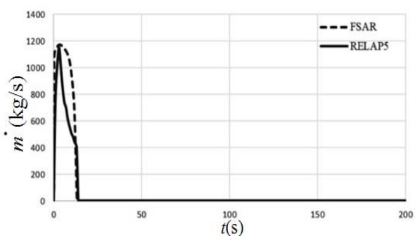
نمودار ۲) میزان دبی شکستگی از سمت اتصال به هدر اصلی بخار
