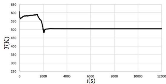
نمودار ۹) دمای سیال خروجی از قلب راکتور برحسب زمان
