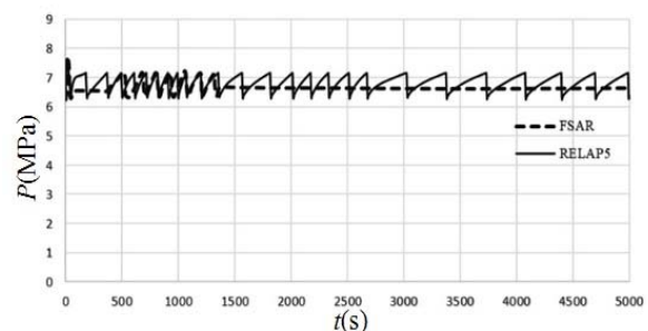
نمودار ۱۲) فشار مولدهای بخار ۱، ۳ و ۴ در ۵۰۰۰ ثانیه اول حادثه
