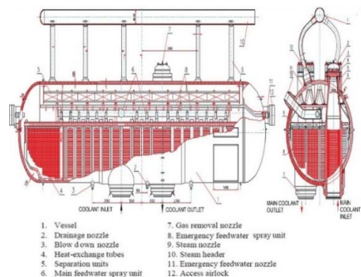
شکل ۱) شماتیک مولد بخار بوشهر [10]
