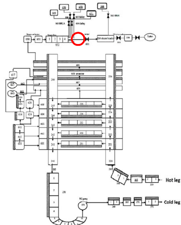
شکل ۳) گره بندی مولد بخار و شاخه های سرد و گرم متصل به آن
