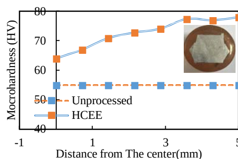
نمودار ۵) توزیع میکروسختی در عرض نمونه منیزیم AM60 اولیه و فرآیندشده توسط فرآیند HCEE
