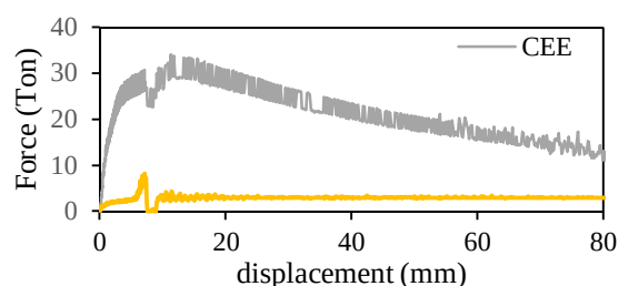
نمودار ۱) مقایسه نیروی لازم برای انجام فرآیند در دو حالت هیدرواستاتیک (HCEE) و سنتی (CEE)
