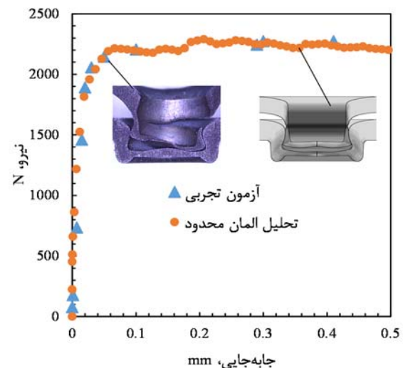
نمودار ۹) نمودار مقایسه استحکام کششی F اتصال سرد حاصل از تحلیل المان محدود و آزمون تجربی در ناحیه قبل از گلوپی شدن
