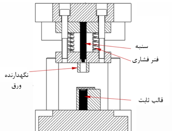
شکل ۵) ابزار طراحی شده برای انجام فرآیند اتصال سرد
