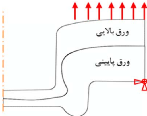
شکل ۳) مدل سازی المان محدود برای تعیین استحکام کششی اتصال سرد بعد از گام شکل دهی اتصال سرد
