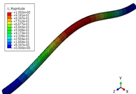
شکل ۱۳) مدلسازی آباکوس کمناش ستون آلومینیومی تقویت شده با کامپوزیت شیشه/ اپوکسی
