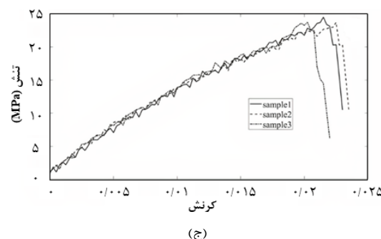
شکل ۸ نمودارهای تنش-کرنش نمونه‌های کامپوزیت اپوکسی/الیاف شیشه، الف: سه نمونه با چیدمان [۰۳]، ب: سه نمونه با چیدمان [۴۵۳]، ج: سه نمونه با چیدمان [۹۰۳]
