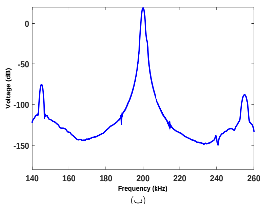
نمودار ۵) طیف پاسخ سازه به اعمال تحریک‌های پمپی (۴۰ کیلوهرتز) و حامل (۲۰۰ کیلوهرتز) حاصل از تحلیل المان محدود؛ الف) حالت سالم، ب) حالت معیوب
