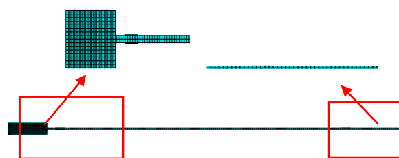
شکل ۳) نحوه گسسته‌سازی تیر، وصله‌های پیزوالکتریک و تکیه‌گاه گیردار
