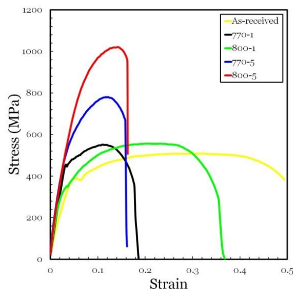
شکل ۱۰) منحنی‌های تنش-کرنش مهندسی فولاد خریداری شده و فولادهای دوفازی تولید شده
