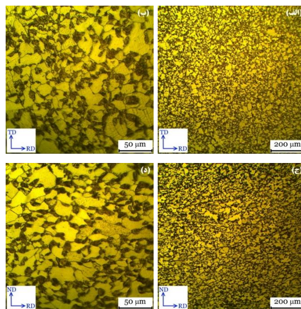
شکل ۶) تصاویر میکروسکوپ نوری در دو صفحه RD-TD و RD-ND فولاد دوفازی تولید شده در دمای 800^{\circ}\text{C} و زمان ۵ دقیقه در دو بزرگ‌نمایی مختلف
