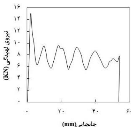
شکل ۱۴) نمودار نیرو بر حسب جابجایی برای نمونه ترکیبی آلومینیوم/کامپوزیت با درصد هم‌پوشانی ۵ درصد.
