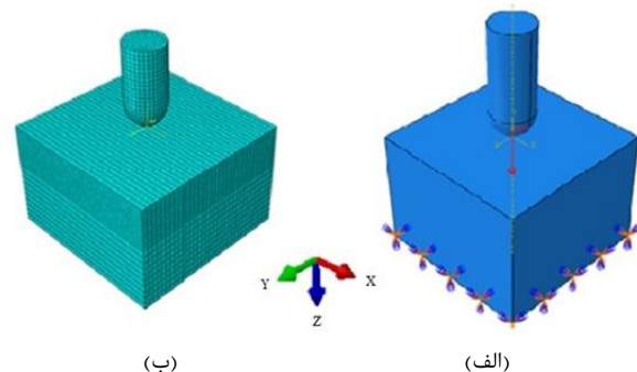
شکل ۷) مدل اجزاء محدود پین و نمونه: (الف) نمایی از پین و نمونه به همراه نقطه مرجع و شرایط مرزی، (ب) نمایی از نحوی مش‌بندی پین و نمونه
