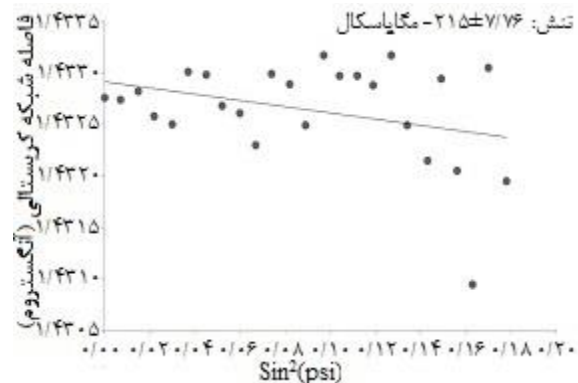
شکل ۶) نمودار فاصله صفحات بلورین بر حسب \sin^2\psi
