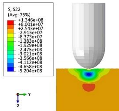
شکل ۸) کانتور تنش پسماند پس از برخورد پین با سطح نمونه
