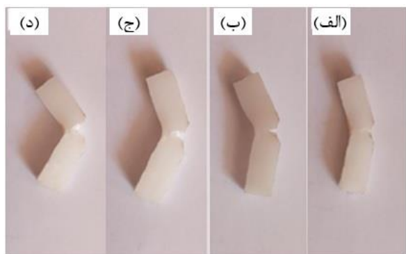
شکل ۵) نمونه‌های تست شاری: الف) HDPE خالص، ب) ۱٪ ZnO، ج) ۳٪ ZnO و د) ۵٪ ZnO
