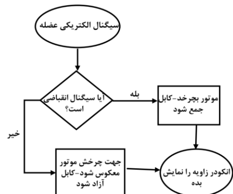
شکل ۵) فلوچارت کنترل با کمک سیگنال زیستی
