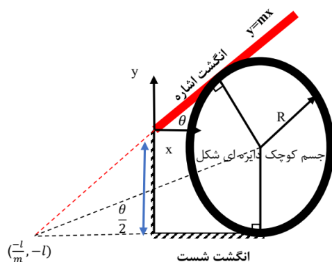
شکل ۶) محاط شدن جسمی به شعاع R بین انگشتان
