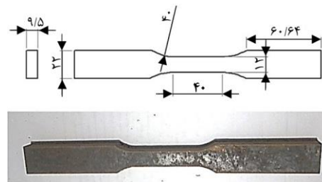
شکل ۵ ابعاد نمونه‌های آزمون خستگی و نمونه آزمون خستگی برش داده شده توسط واترجت
