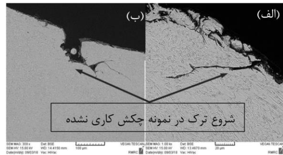
شکل ۸) تصویر میکروسکوپ الکترون روبشی نشان‌دهنده ترک در نمونه چکش کاری نشده با بزرگنمایی (الف) ۳۰۰ و (ب) ۱۰۰۰ برابر
