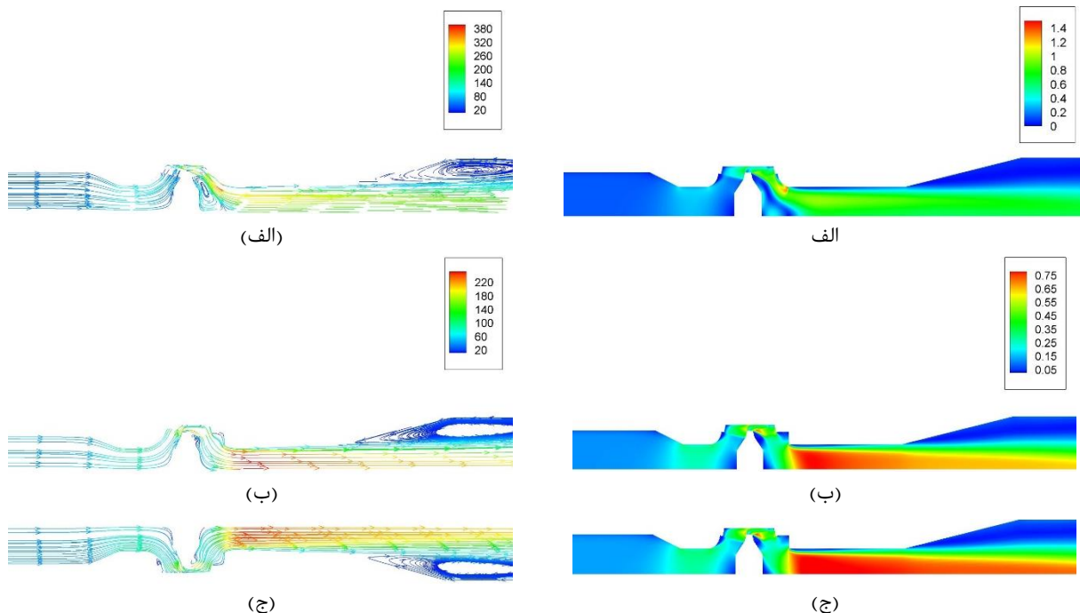
شکل ۱۰) تغییرات عدد ماخ برای شرایط الف) بدون ساینسر، ب) با ساینسر ۱۰ ppi، ج) با ساینسر ۲۰ ppi شکل ۱۱) خطوط جریان رنگی شده با اندازه سرعت (m/sec) برای شرایط الف) بدون ساینسر، ب) با ساینسر ۱۰ ppi، ج) با ساینسر ۲۰ ppi
