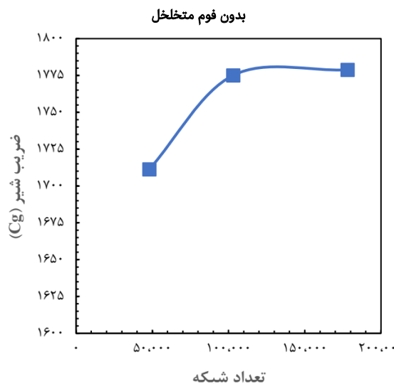
شکل ۶ بررسی استقلال از شبکه برای رگلاتور بدون سایلنسر
