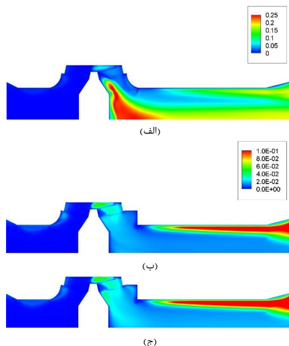
شکل ۱۴ تغییرات ویسکوزیته تلاطم (kg/m/sec) برای شرایط الف) بدون ساینس، ب) با ساینس ۱۰ ppi، ج) با ساینس ۲۰ ppi
