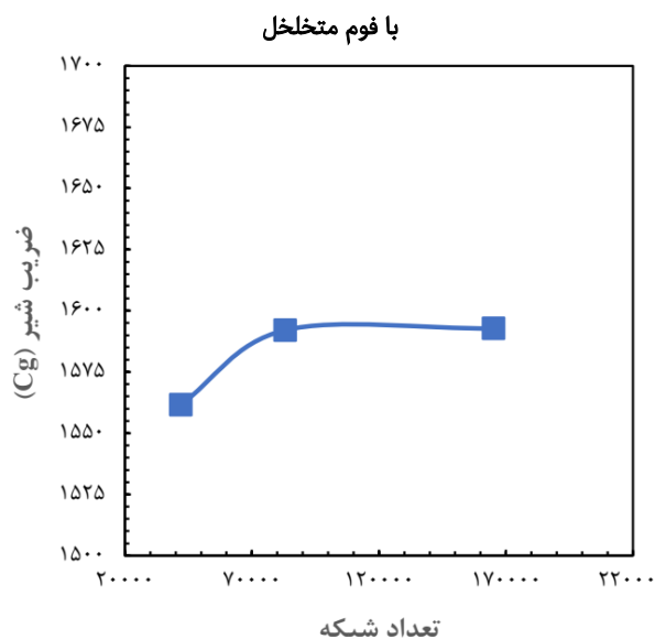
شکل ۷ بررسی استقلال از شبکه برای رگلاتور با سایلنسر
