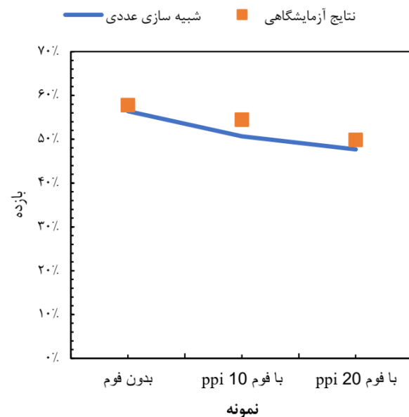
شکل ۹) نمودار تغییرات بازده در شرایط مورد بررسی
