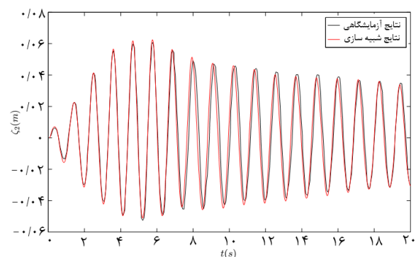
شکل ۱۱) تجزیه‌ی آزاد امواج متلاطم. مقایسه‌ی بین نتایج عددی و آزمایشی [9] برای ارتفاع موج در فاصله‌ی ۵ میلی‌متری از دیواره‌های عمودی به ازای h/l = 883/0, \eta_{2a} = 0.0465/m, \omega/\omega_1 = 1/1 . حرکت عرضی اجباری در زمان ۷/۴ ثانیه متوقف می‌شود.
