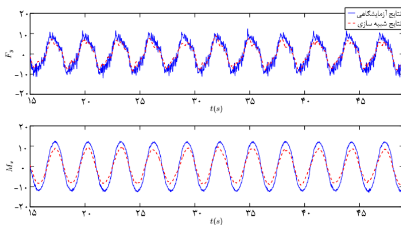
شکل ۶) مقایسه‌ی نتایج آزمایشگاهی و عددی نیروی عرضی و ممان رول در تست ۲۰ و \frac{\omega}{\omega_1} = 1/10, \phi_a = 4/10^\circ
