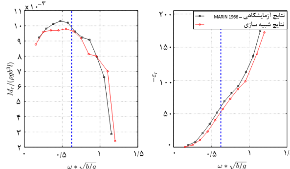
شکل ۱۶) مقایسه‌ی نتایج آزمایشگاهی و عددی ممان رول (سمت چپ: دامنه بدون بعد ممان. سمت راست: اختلاف فاز) حول محور چرخش به ازای \phi_a = 9/10, h/b = 0.4, s = 0 . خط چین آبی، فرکانس طبیعی اسلاشینگ بصورت تئوری را نشان می‌دهد.
