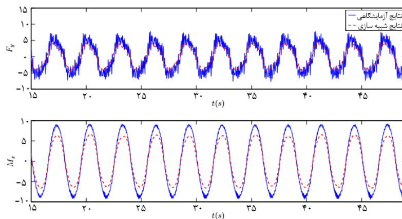
شکل ۷) مقایسه‌ی نتایج آزمایشگاهی و عددی نیروی عرضی و ممان رول در تست ۳۰ و \frac{\omega}{\omega_1} = 1/10, \phi_a = 2/10^\circ
