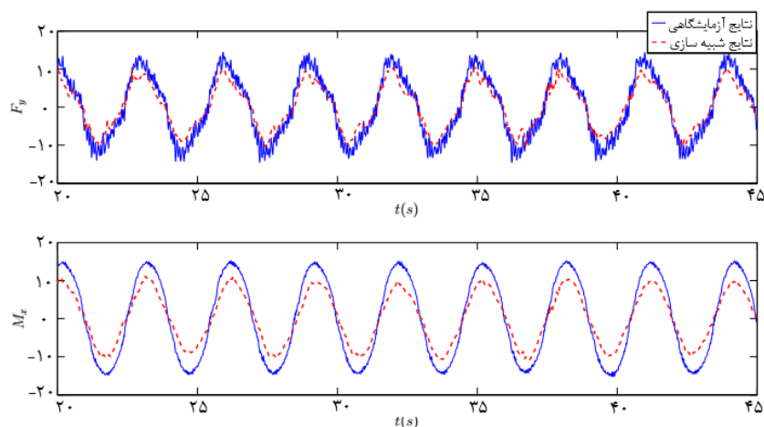
شکل ۵) مقایسه‌ی نتایج آزمایشگاهی و عددی نیروی عرضی و ممان رول در تست ۰۶ و \frac{\omega}{\omega_1} = 1/10, \phi_a = 6/10^\circ
