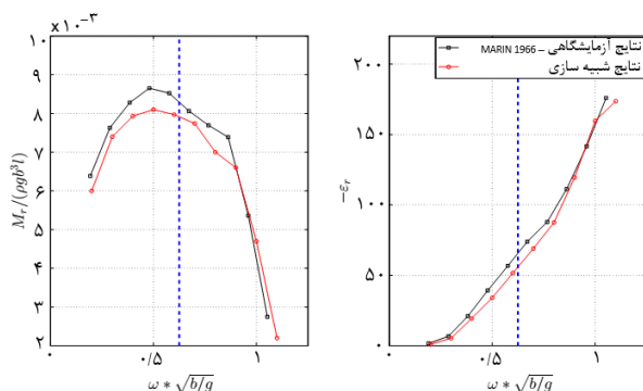
شکل ۱۳) مقایسه‌ی نتایج آزمایشگاهی و عددی ممان رول (سمت چپ: دامنه بدون بعد ممان. سمت راست: اختلاف فاز) حول محور چرخش به ازای \phi_a = 9/10, h/b = 0.4, s = 0 . خط چین آبی، فرکانس طبیعی اسلاشینگ بصورت تئوری را نشان می‌دهد.
