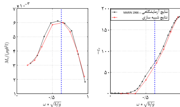
شکل ۱۴) مقایسه‌ی نتایج آزمایشگاهی و عددی ممان رول (سمت چپ: دامنه بدون بعد ممان. سمت راست: اختلاف فاز) حول محور چرخش به ازای \phi_a = 7/5, h/b = 0.4, s = 0 . خط چین آبی، فرکانس طبیعی اسلاشینگ بصورت تئوری را نشان می‌دهد.
