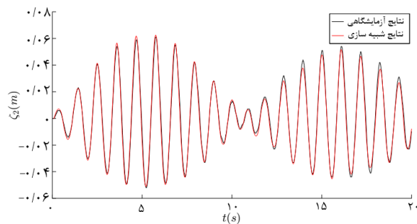
شکل ۱۰) مقایسه‌ی بین نتایج آزمایشگاهی و عددی برای ارتفاع موج در فاصله‌ی ۵ میلی‌متری از دیواره‌های عمودی برای h/l = 883/0, \eta_{2a} = 0.0465/m, \omega/\omega_1 = 1/1
