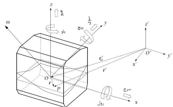
شکل ۳) دستگاه مختصات ثابت بدنه (Body-fixed coordinate system) مورد استفاده در حلگر اسلاشینگ [10].
