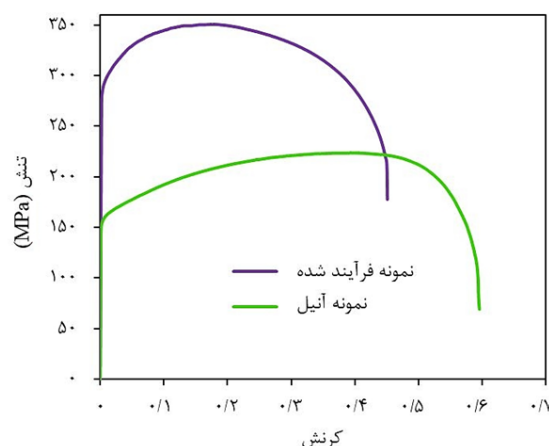
شکل ۶) نمودار تنش مهندسی-کرنش مهندسی حاصل از آزمون کشش برای نمونه‌ی آنیل فرآیند نشده و نمونه‌ی یک مرحله فرآیند اکستروژن شدن فشاری تناوبی هیدرواستاتیک لوله شده
