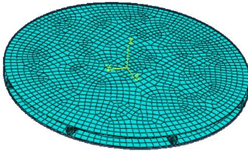
شکل ۵) مدل اجزاء محدود سازه
