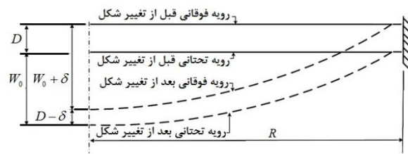
شکل ۲) هندسه نیمی از مقطع سازه قبل و بعد از تغییر شکل
