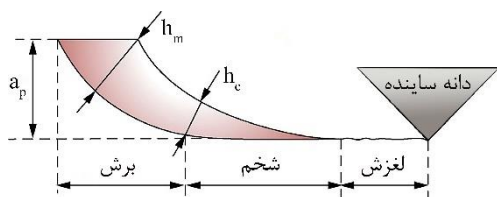
شکل ۱) میکرو مکانیزم‌های براده‌برداری بین دانه ساینده و قطعه کار [12]
