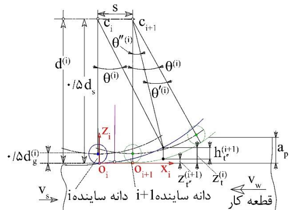
شکل (۴) آنالیز سینماتیکی مسیر حرکت چندین دانه ساییده
