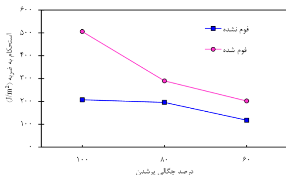
شکل ۵) نتایج استحکام به ضربه نمونه‌های فوم نشده و فوم شده در درصد‌های بر شدن متفاوت
