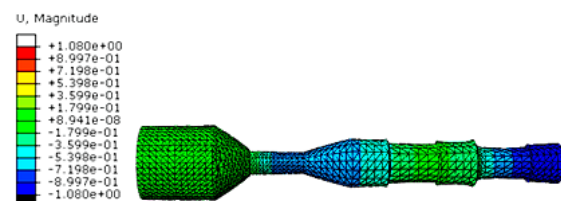
شکل ۹) نمایش فرکانس طبیعی هورن و شکل مود طولی مدل نهایی
