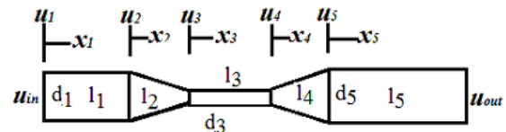
شکل ۴) شماتیک هورن باربل به همراه اندازه
