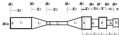
شکل ۸) شماتیک هورن باربل چند پله‌ای
