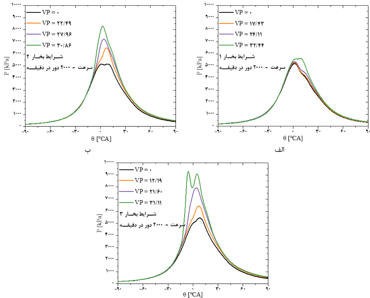
شکل ۱۲) منحنی فشار در سرعت ۲۰۰۰ دور در دقیقه در شرایط با بخار گازوئیل و بدون بخار گازوئیل، (الف) در شرایط بخار ۱، (ب) در شرایط بخار ۲ و (ج) در شرایط بخار ۳
