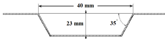
شکل (۱) شماتیک قطعه نهایی
