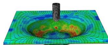
شکل (۴) ورق شکل داده شده در شبیه‌سازی اجزا محدود
