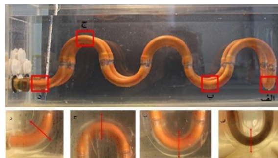
شکل ۸) یخ تشکیل شده در چهار محل از لوله در انتهای آزمایش (الف) ورودی لوله (ب). اولین برآمدگی در مسیر ورودی لوله (ج) فاصله ۴۶ سانتیمتری از ورودی لوله (د) منحنی U شکل انتهای لوله
