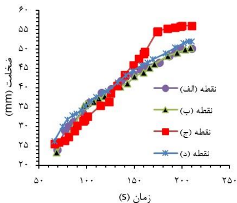
شکل ۶) متوسط ضخامت یخ تشکیل شده نسبت به زمان در چهار محل از لوله در انتهای آزمایش (الف) ورودی لوله (ب). اولین برآمدگی در مسیر ورودی لوله (ج) فاصله ۴۶ سانتیمتری از ورودی لوله (د) منحنی U شکل انتهای لوله
