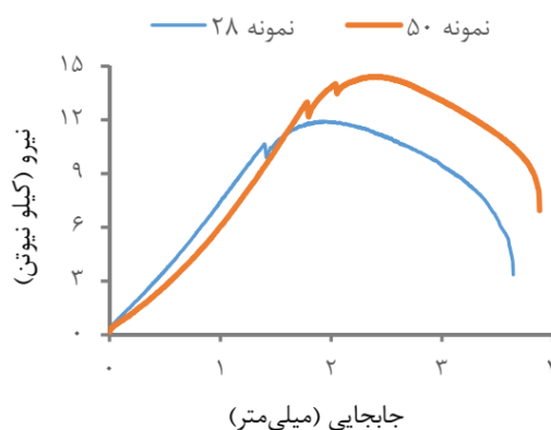
شکل ۱۴) مقایسه نمودار نیرو - تغییر طول برای دو قطعه ترمیم شده با وصله مستطیلی و H شکل (قطعات ۲۸ و ۵۰) و مساحت مؤثر یکسان
