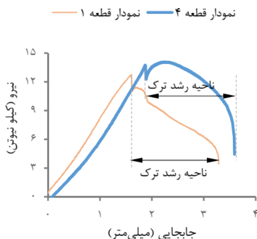
شکل ۷) مقایسه نمودار نیرو- تغییر طول نمونه‌های شماره ۱ و ۴
