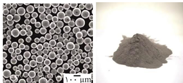
شکل ۲) پودر فولاد ۱۷- PH4 و ریخت‌شناسی ذرات آن
