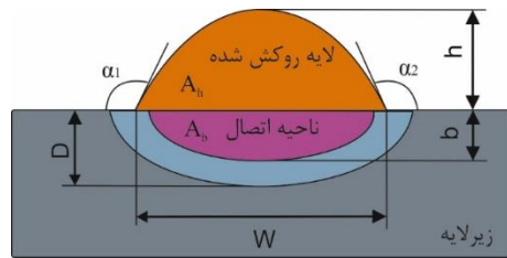
شکل ۵) ترسیمه‌ای از هندسه لایه روکش‌شده در سطح مقطع عرضی
