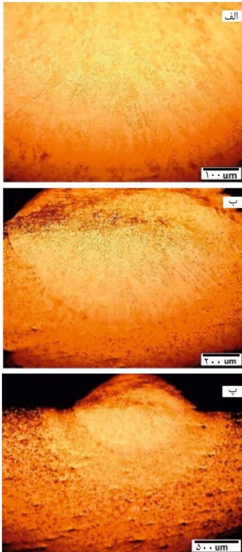
شکل ۶) تصاویر سطح مقطع عرضی نمونه شماره ۱ در سه بزرگنمایی: الف) x20، ب) x10، پ) x5.
