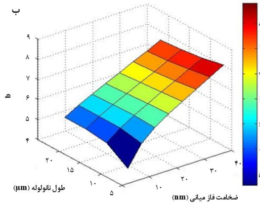
شکل ۷) منحنی‌های تاثیر پارامترهای t و \lambda روی b : الف) دوبعدی و ب) سه بعدی
