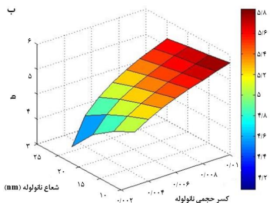
شکل ۶) منحنی‌های تاثیر پارامترهای \varphi_f و R روی b : الف) دوبعدی و ب) سه بعدی
