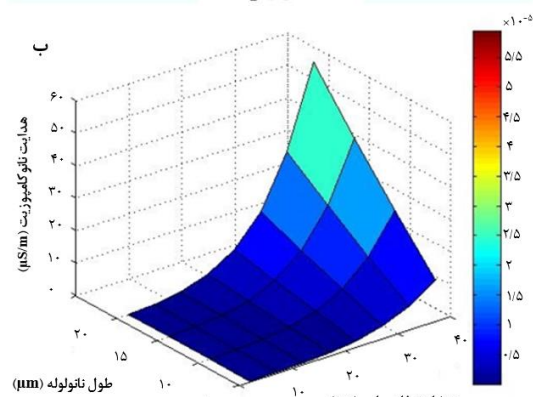
شکل ۸) منحنی‌های تأثیر پارامترهای t و l در \sigma_f : الف) دوبعدی و ب) سه بعدی
