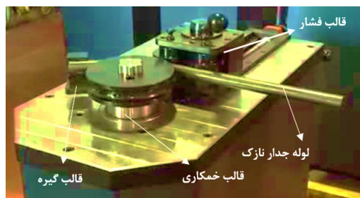
شکل ۱) دستگاه و تجهیزات خمش لوله مورد استفاده در این پژوهش
